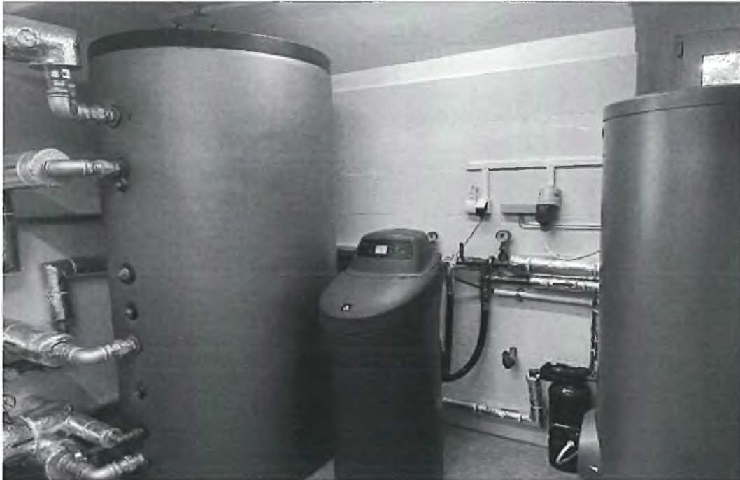
fot. Środowiskowy Dom Samopomocy w Oleśnicy Małej – od lewej strony: Zbiornik Buforowy np.: Reflex HF (2) Stacja demineralizacji wody grzewczej np.:SYR 3200 (1) oraz istniejący podgrzewacz wody 200 l.
